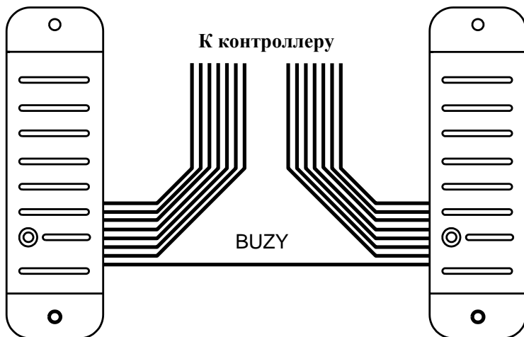
Рис. 2 Схема включения двух рядом расположенных считывателей для устранения их взаимного влияния друг на друга.
