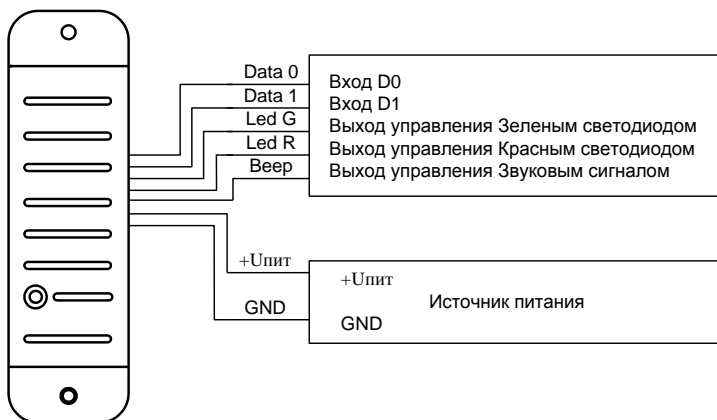
Рис. 1 Схема подключения считывателя к контроллеру с интерфейсом Wiegand (если взаимоблокировка двух считывателей не производится, то провод Buzy – не подключается).
