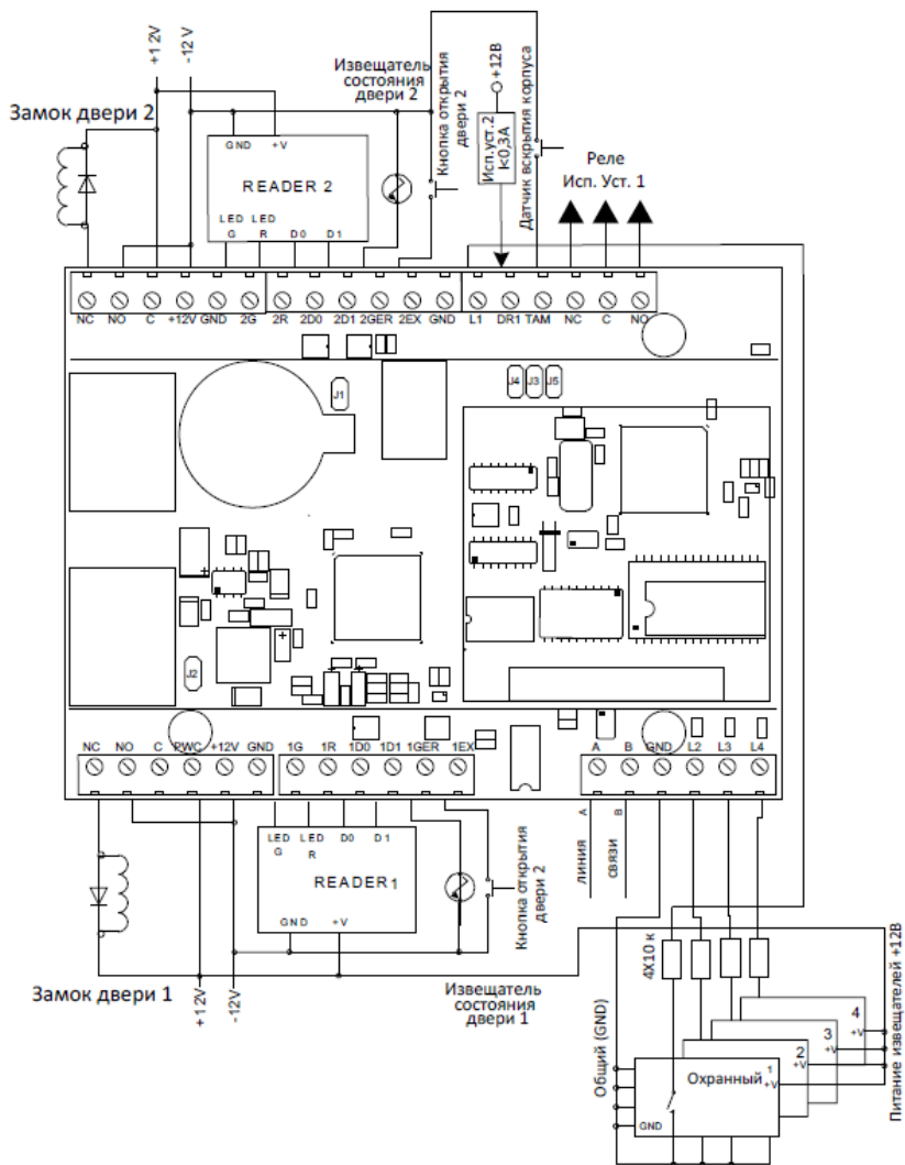
Схема подключения
