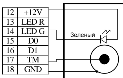
Считыватель с одним индикатором
