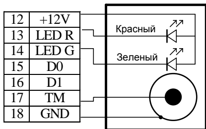
Считыватель с двумя индикаторами
