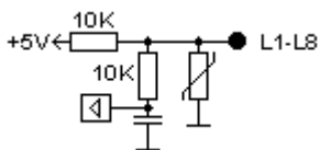
Схема входных цепей L1-L4 контроллера:
