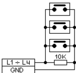
Схема включения с “нормально разомкнутыми контактами”:
